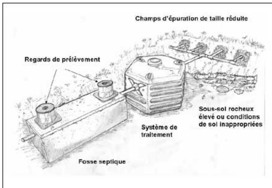
Figure 5 : Autre technique de traitement (Source : Éric Brunet, Centre ontarien des eaux usées rurales, Université de Guelph)
