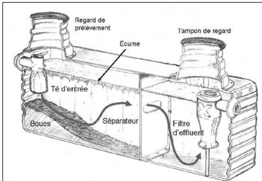
Figure 2 : Vue en coupe d'une fosse septique courante avec regards de prélèvement et filtre d'effluent (Source : Éric Brunet, Centre ontarien des eaux usées rurales, Université de Guelph)
